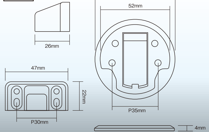
寸法図
